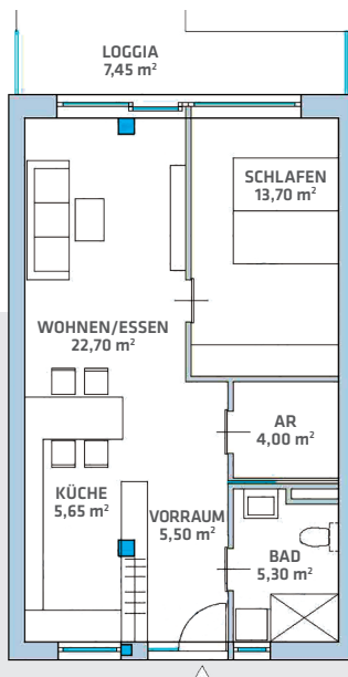
Grundriss 60 m 2 Einzelwohnung
